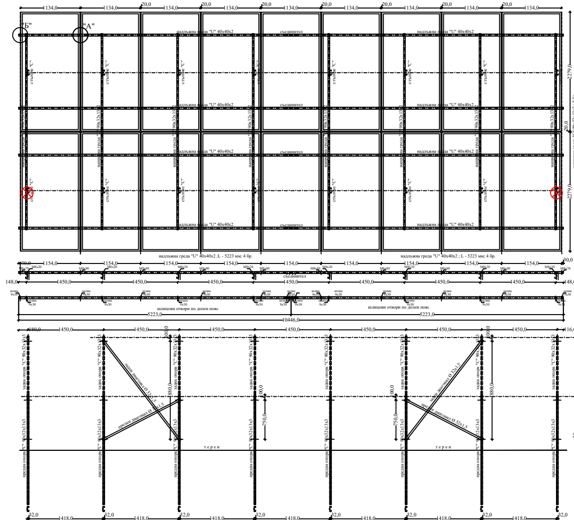
МОНТАЖЕН ПЛАН - модулна метална конструкция за монтаж portrait на 2 реда х 9 бр. PV(2279x1134x35), ъгъл 30°
